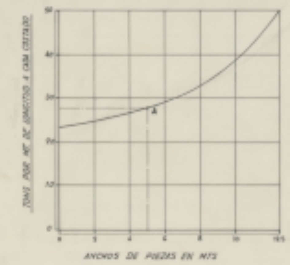
GRAFICO PARA CARGAS PESADAS
